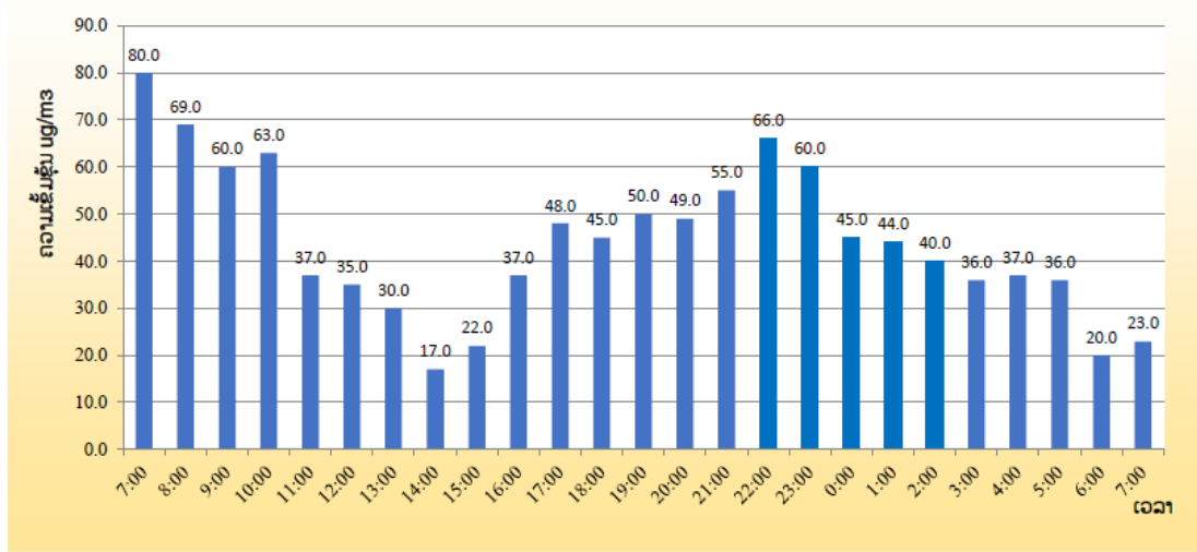
ຜົນການວັດແທກປະລິມານຜຸ່ນລະອອງ PM 2.5 ເປັນແຕ່ລະຊົ່ວໂມງໃນ ວັນທີ 21- 22 ເມສາ 2020 ບ້ານ ຊຽງຍົນ (ສວນເຈົ້າອານຸວົງ )
