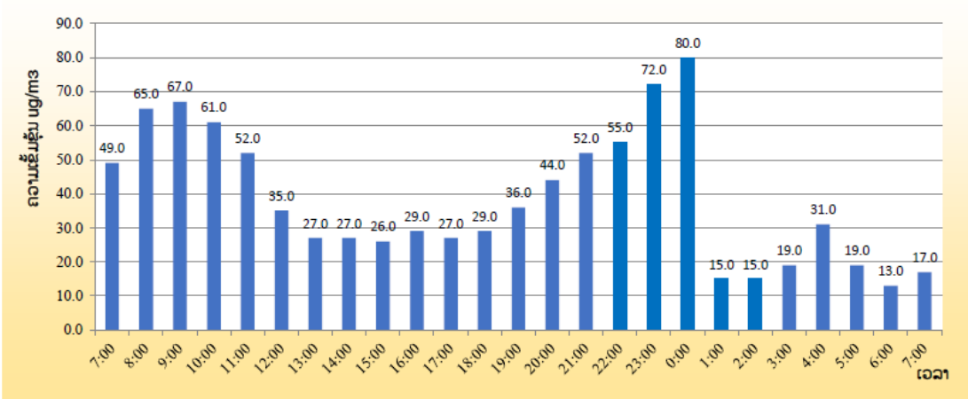
ຜົນການວັດແທກປະລິມານຝຸ່ນລະອອງ PM 2.5 ເປັນແຕ່ລະຊົ່ວໂມງໃນ ວັນທີ 21- 22 ເມສາ 2020 ບ້ານ ໂນນທອງ (ອຸດສາຫະກຳຫຼັກ 21)
