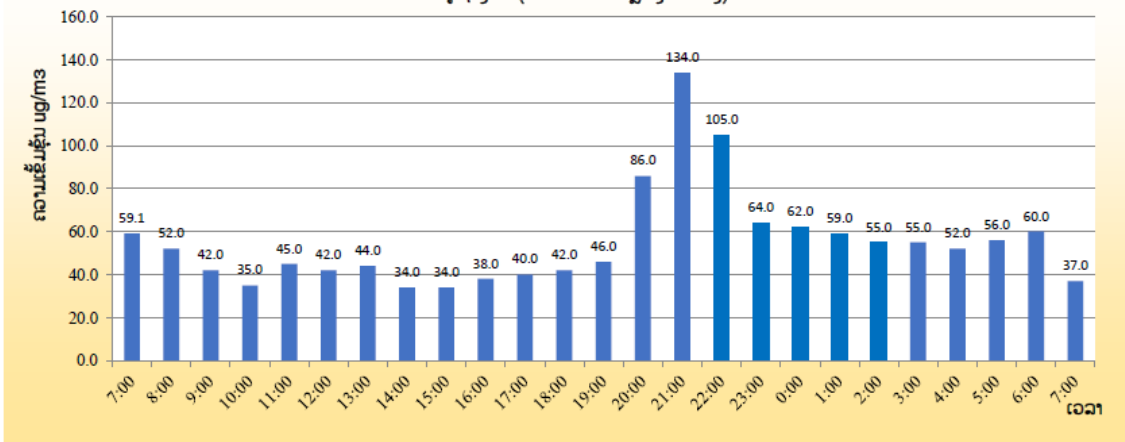
ຜົນການວັດແທກປະລິມານຝຸ່ນລະອອງ PM 2.5 ເປັນແຕ່ລະຊົ່ວໂມງໃນ ວັນທີ 21- 22 ເມສາ 2020 ບ້ານ ພູຊ້າງຄໍາ (ສະໜາມບິນຫຼວງພະບາງ)
