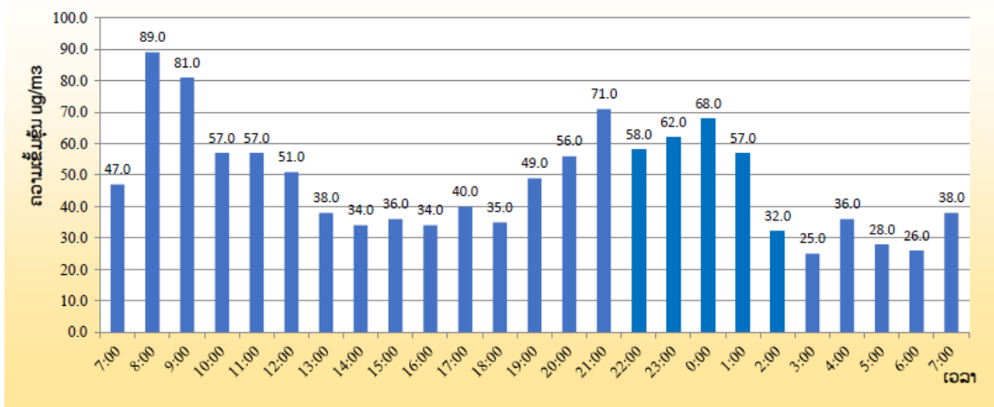
ຜົນການວັດແທກປະລິມານຝຸ່ນລະອອງ PM 2.5 ເປັນແຕ່ລະຊົ່ວໂມງໃນ ວັນທີ 21- 22 ເມສາ 2020 ບ້ານ ໂນນສະອາດ (ດົງໝາກຄາຍ)
