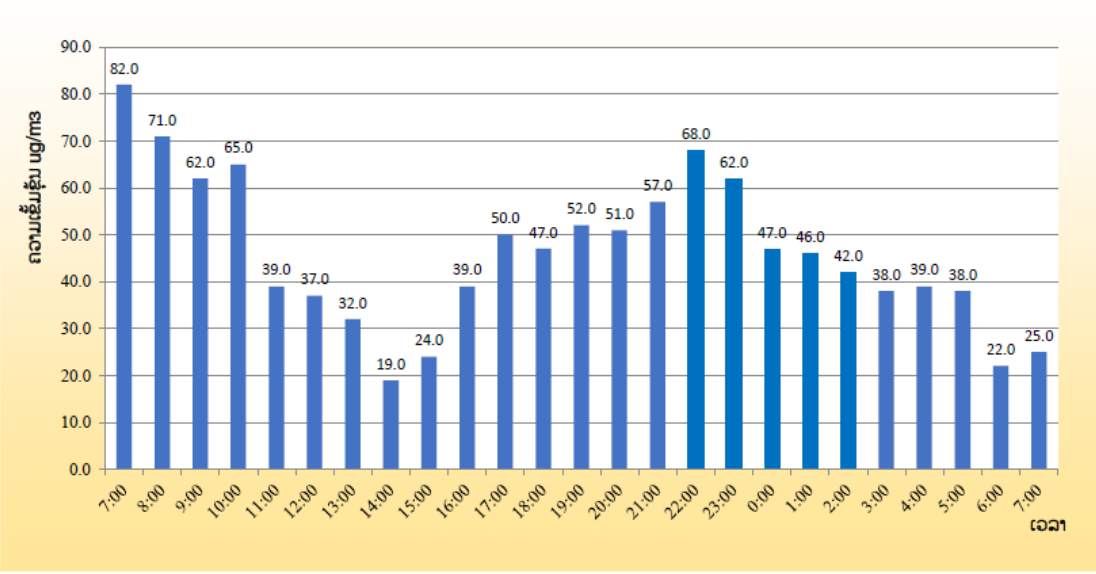
ຜົນການວັດແທກປະລິມານຜຸ່ນລະອອງ PM 2.5 ເປັນແຕ່ລະຊົ່ວໂມງໃນ ວັນທີ 21- 22 ເມສາ 2020 ບ້ານ ອາກາດ (ກົມອຸຕຸນິຍົມ ແລະ ອຸທິກກະສາດ )
